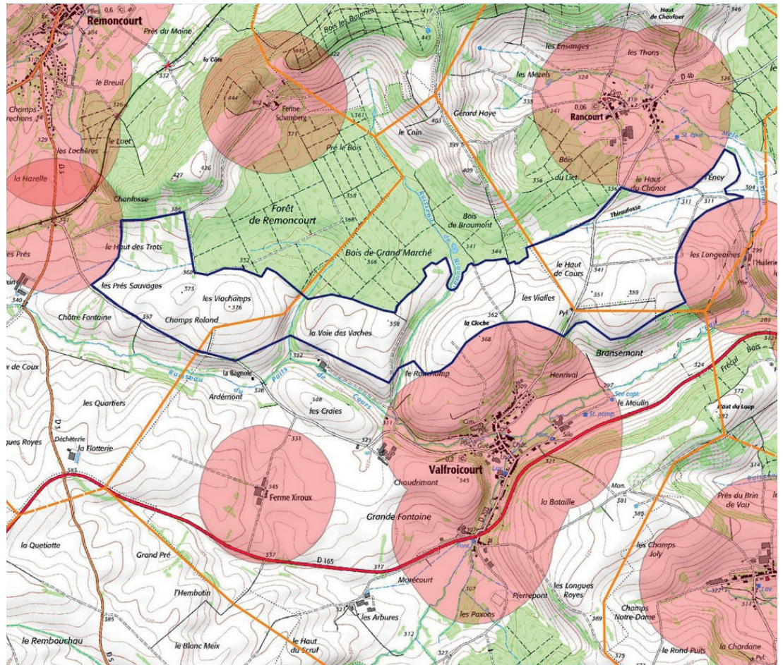
Carte de la zone d'implantation provisoire du projet éolien, avec identification des contraintes liées aux habitations.
